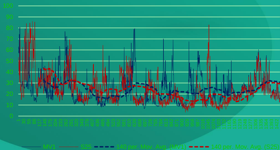
Srovnání průběhu 10 min. koncentrací NO 2
