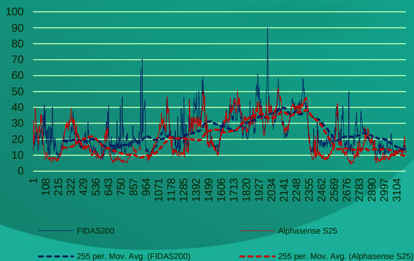
Srovnání průběhu 5 min. koncentrací PM10
